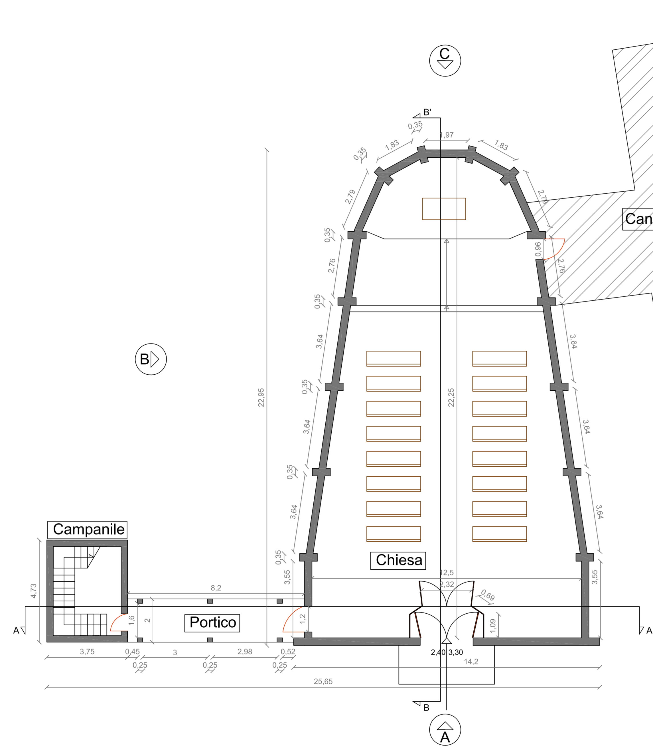
Pianta quota 0,50 m Scala 1:100
