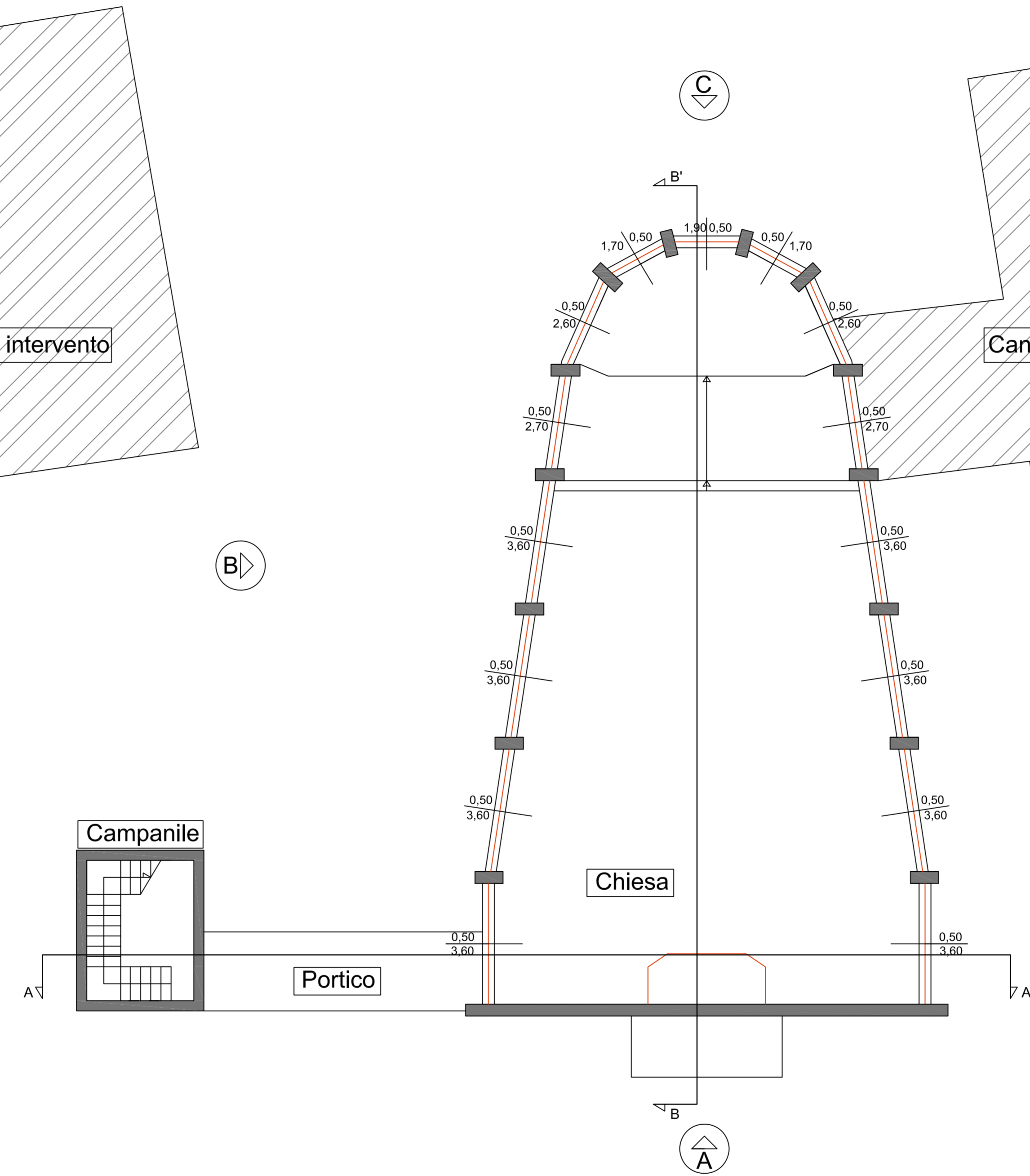
Pianta quota 4,80 m Scala 1:100
